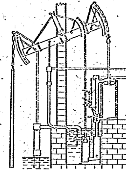
第五圖 ワットノ單動機關
