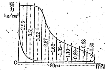
第九圖 指壓線圖ノ一例
