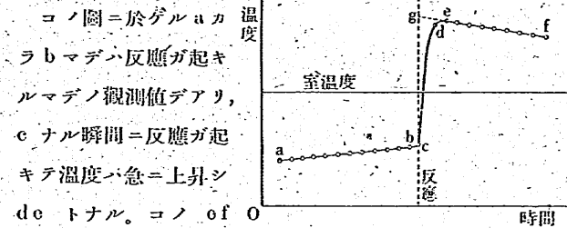
第二圖 溫度計ノ讀ミノ時間的變化
