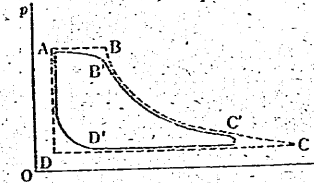
第八圖 指壓線圖 ABCD ハ標準循環過程、 AB'C'D' ハ實際ノ循環過程
