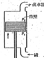
第六圖 雙動シリンダ
