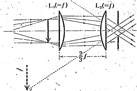
第二十六圖 接眼鏡
