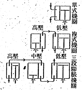
第十五圖 多段膨脹機關
