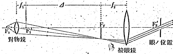
第二十四圖 顯微鏡
