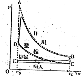
第十六圖 四行程定容サイクル
