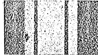
第四十六圖 一木ノ細隙ノ回折ニヨル干渉縞
