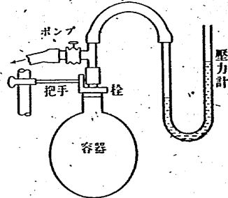
第十一圖 比熱比ノ測定装置
