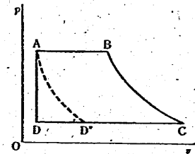
第十四圖 蒸氣機關ニ於ケル水ノ理想的ナ循環過程 ABCD トカルノー・サイクル ABCD'
