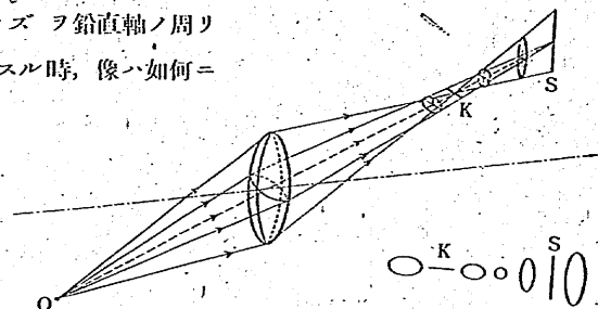
第三十圖 光軸上ニナイ物點ノ作ル二種ノ焦點
