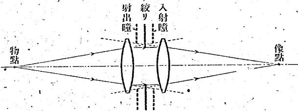
第二十二圖 寫真レンズ
