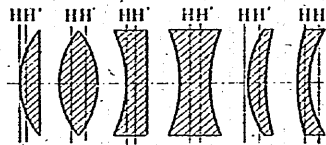
第三十七圖 種々ノレンズノ主點ノ位置
