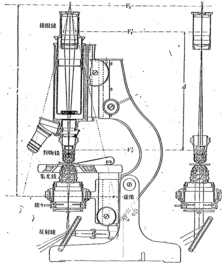
アボクロマト顯微鏡ノ最新シイ型式ノウツ集光鏡ガ非常ニ複雑ニデキテアル。 l ハ明視距離、 D ハ對物鏡ノ後焦點 F_1 、ト接眼鏡ノ前焦點 F_2' トノ距離デアアル。
