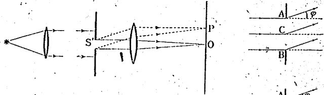
第四十四圖 一木ノ細隙ニヨル光ノ干渉
