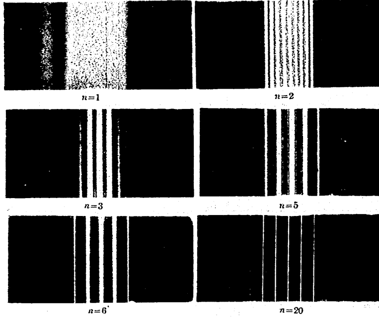
平行ナ細隙ニヨル光ノ回折縞 (n ハ細隙ノ數)
