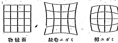
第三十三圖 碁盤目ノ像ノユガミ
