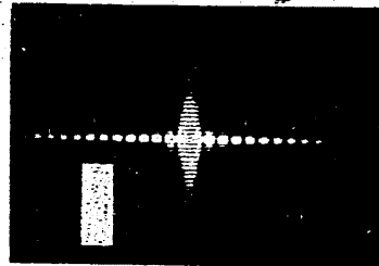
第四十八圖 板體ノ影ノ縁ニ生ズル干渉縞
