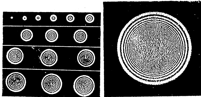
點光源カラノ光ガ種々ノ大キサノ圓孔ニヨツテ生ジタ回折ノ輪
