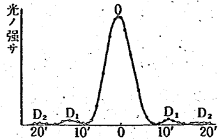
第四十七圖 矩形ノ孔ノ作ル干渉縞
