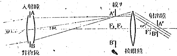
第二十五圖 凸レンズ望遠鏡
