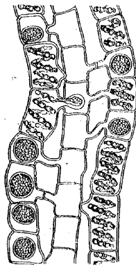
図4 アオミドロ
