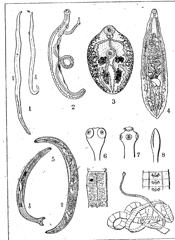
図 2. 寄生虫
