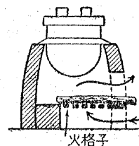
第 28 図 かまど (3)
