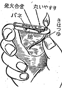
第44図 ライトターの構造
