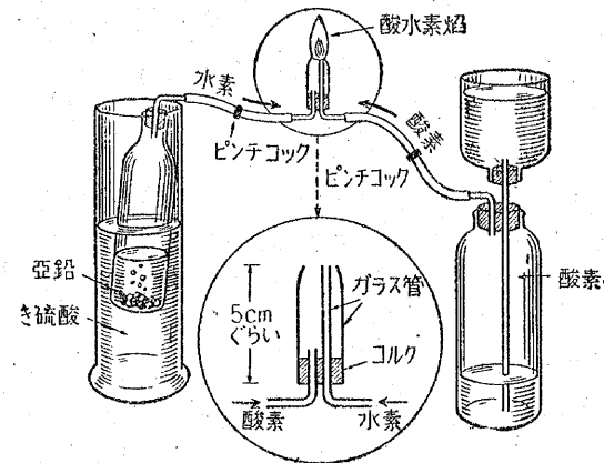
第 40 図 実験 14. 酸素水素焰
