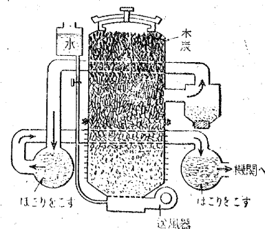
第3図 乗合自動車の木炭ガス発生炉
