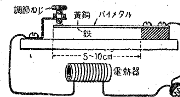
第21図 サーモスタット
