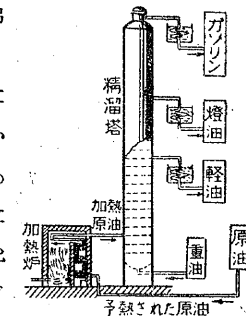
第18図 原油からガソリン・燈油・軽油を分けとるしかけ
