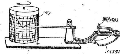
第20図 自記温度計
