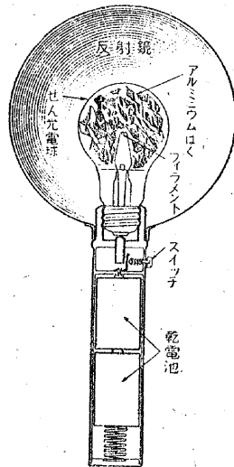
第10図 セン光電球
