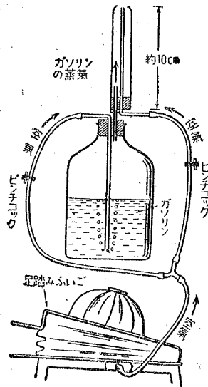
第 38 図 エアガス装置
