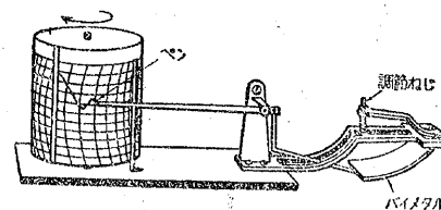
第20図 自記温度計
