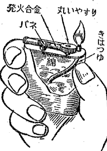
第44図 ライターの構造
