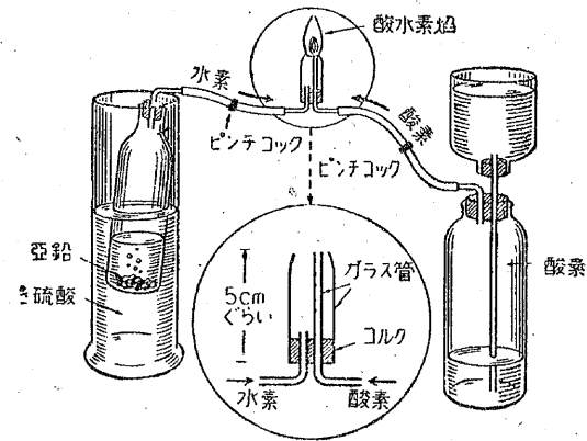
第 40 図 実験14. 酸素アセチレン焰
