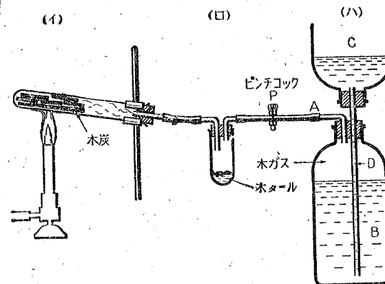
第13図 実験9のしかけ
