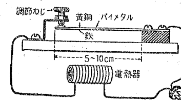
第21図 サーモスタット
