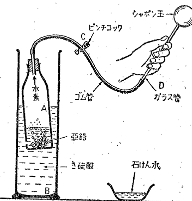
第4図 実験4の装置
