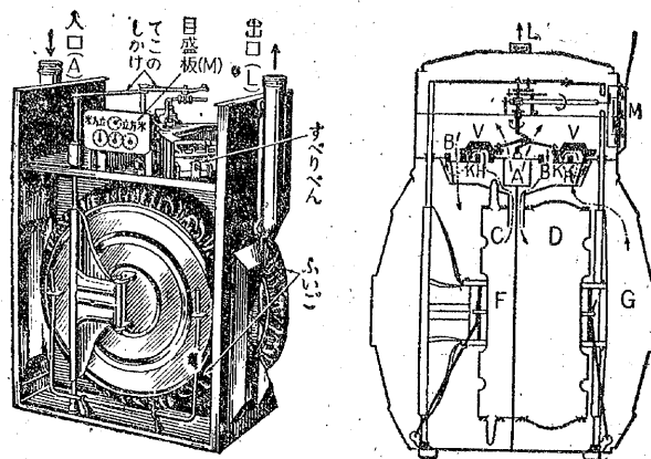
第34図 ガスメーター
