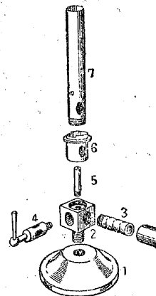
第35図 ガスバーナー
