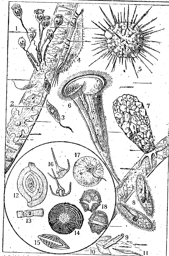
1. つりがねむし 2. アメーバ 3. みどりむし 4. スチロキア 5. たいよう ちゅう 6. らっぱむし 7. ディフルギア 8. ぞうりむし 9. 10. 11. けいそう 12. 13. 14. 15. 有孔虫 16. ケラチウム 17. 夜光虫 18. ペリジニウム 1.—11. 淡水にすむ原生生物 12.—18. 海水にすむ原生生物
