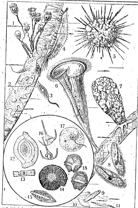
1. つりがねむし 2. アメーバ 3. みどりむし 4. スチロキア 5. たいよう ちゅう 6. ろっぱむし 7. ディフルギア 8. ぞうりむし 9. 10. 11. けいそう 12. 13. 14. 15. 有孔虫 16. ケラチウム 17. 夜光虫 18. ペリジニウム 1.—11. 淡水にすむ原生生物 12.—18. 海水にすむ原生生物
