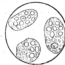
アメーバ赤痢の病原体 (約 200 倍)
