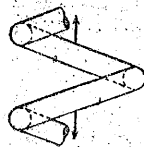
第37図 つる巻き ばねの棒のねじれ を示す。わかりや すいために途中を (じっさいには曲 がっているが) 直 線で表わしている。
