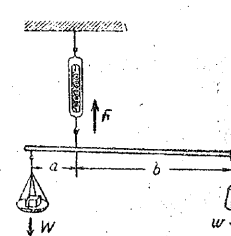
第 25 図 さおばかりのつり合
