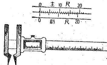
第 61 図 ノギスと副尺
