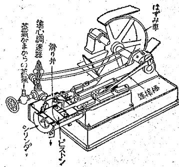
第114図 蒸気機関
