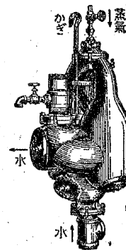
第97図 だるまポンプ とくり のよ うな器が2箇あ り、交互に水を 吸いこみ蒸気で 押し上げる。か き は使うとき に上からつるす ためのものでは ある。
