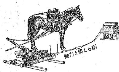
第10図 畜力原動機
