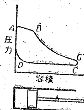
第116図 指圧線図
