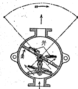
第92図 ウィングポンプ
