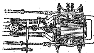
第123図 ルノーアルのガス機関
