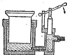
第98図 水圧機
