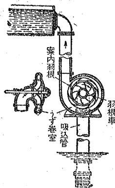
第96図 (a) うず巻ポンプ べるフランスス水車に似ているので、タービンポンプともいう。案内羽根を使わない場合もそうとうに多い。このポンプは、わりあいに低い所にたくさんの水
