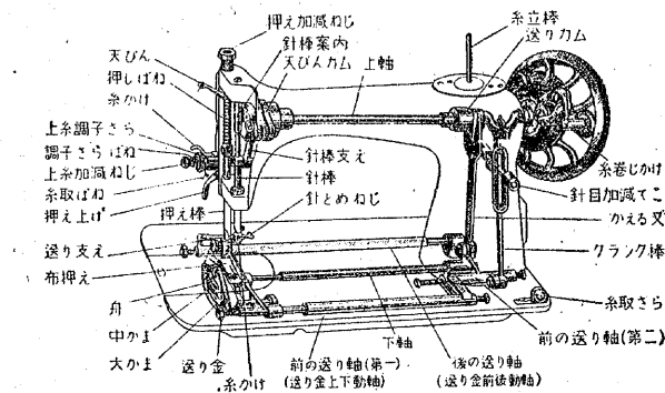
第 107 図 ミ シ ン
