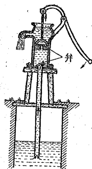
第91図 吸上げポンプ
