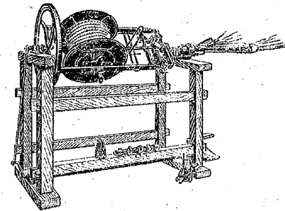
第9図 足踏みなわなない機
