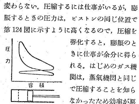
第124図 内燃機関指圧線図
