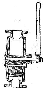
第92図 ウィングポンプ
