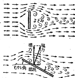
第81図 揚力と抵抗
