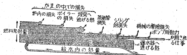
第115図 蒸気機関の熱の行ぐえ
