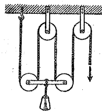
第 24 図 組合せ滑車
