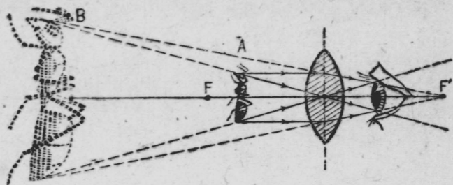
第9図 虫めがね。物を焦点Fのすぐうしろへおくと、光はレンズを通してから開いて、Bから来たように見える。
