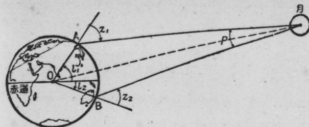
第16図 同一子午線上の2点A, Bから同時に月を観測して、その天頂距離 Z_1, Z_2 を測定する。A, Bの緯度が南北に l_1, l_2 とすると、 P = (Z_1 + Z_2) - (l_1 + l_2) となる。
