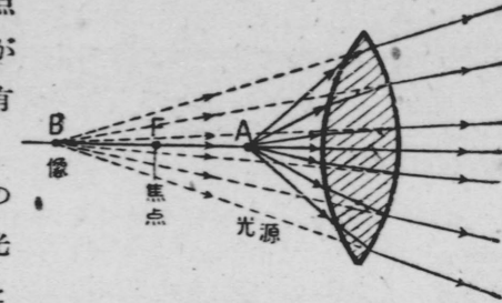
第8図 Aから出た光線はBに光源をおいたときと同様に進む。Bを"虚像"という。
