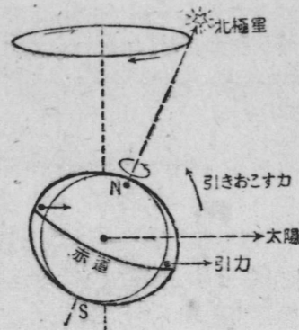
第37図 地球の歳差運動
