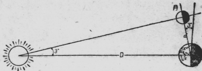
第 18 図 アリストタルコスの方法
