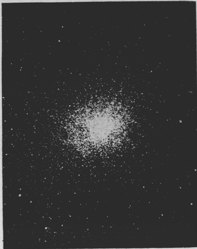
附 図 7 球状星団（ヘルクレス星座）
