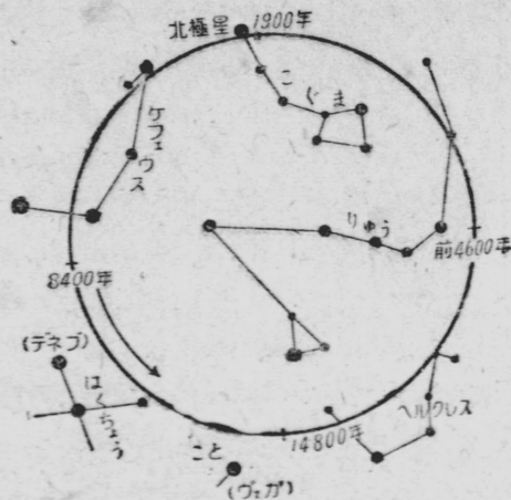
第38図 天球の北極の移動
