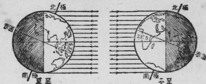
第28図 夏至と冬至のときの太陽光線のあたりかた。
