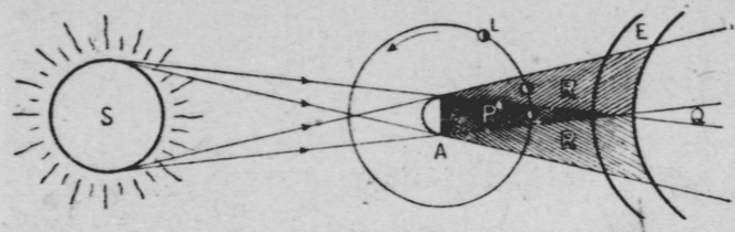
第33図 日食・月食のおこるわけ。Aを地球とすればLを月とみてよい。Aを月とみればEが地球になる。
