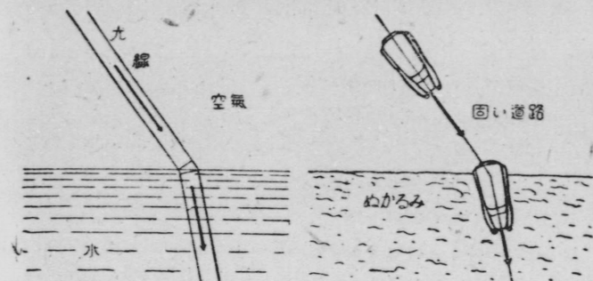
第3図 ぬかるみに落ちこんだ自動車と光線の屈折。
