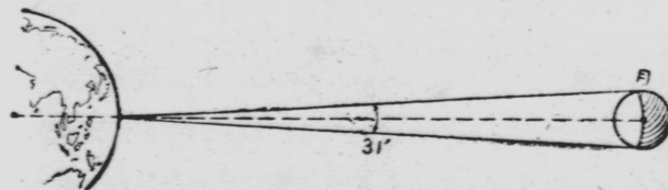
第17図 月までの距離がわかれば、月の半径がわかる。
