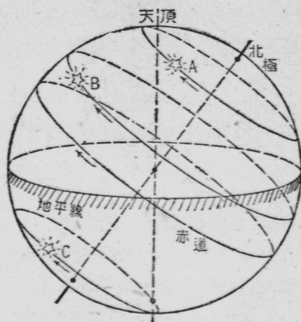
第40図 毎日東から西へ回轉する天球。
