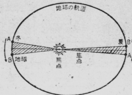
第29図 地球の軌道は正しくはダエン形で、太陽はその一方の焦点にいる。
