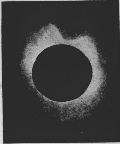
第24図 1919年の日食の際のコロナ。
