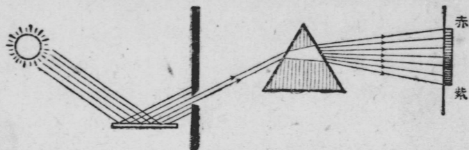
第25図 太陽光線の連続スペクトルをとること。ニュートンはこうして光をしらべた。
