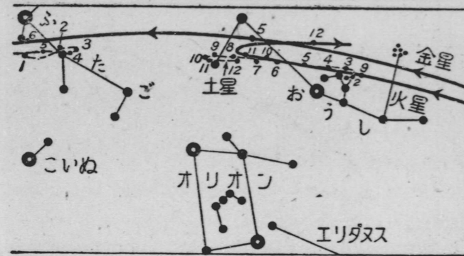
惑星の運動
