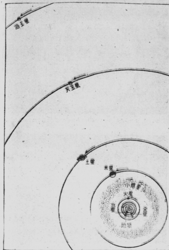
第20図 太陽系の諸惑星とその軌道
