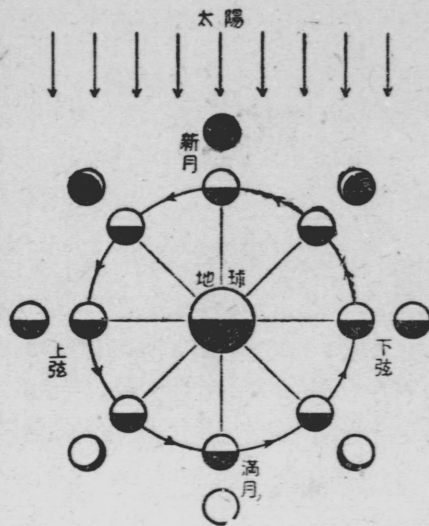
第32図 月の満ち欠け
