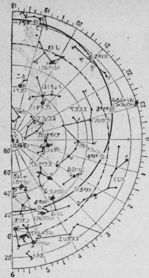
北天の星座
