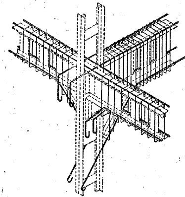
第47図 鉄骨・鉄筋コンクリート造
