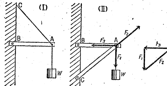
第43図 一端が自由なはりの補強
