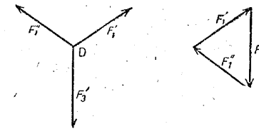
第40図 D点に働く力
