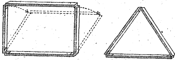
第29図 四角形の組合せと三角形の組合せ
