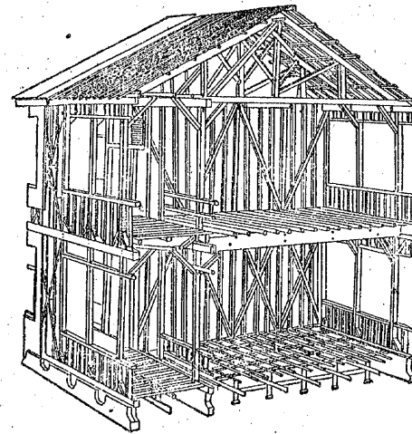
校舎の骨組
