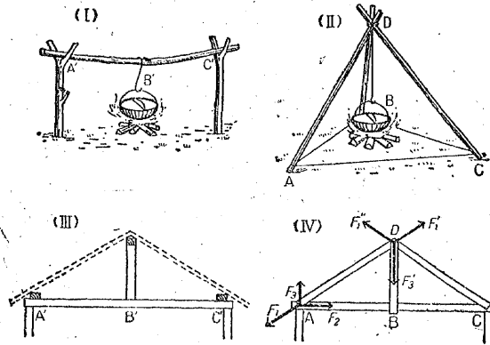
第39図 はりの補強
