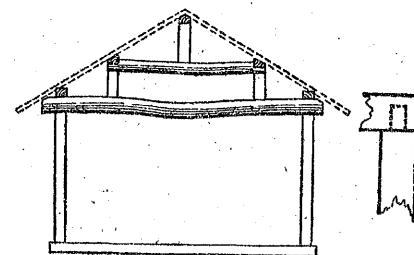
第33図 和小屋の骨組
