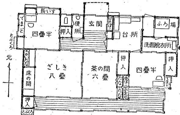
第49図 住宅の平面図
