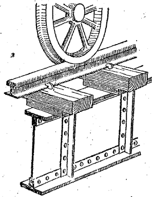
第25図 鋼板橋とレール
