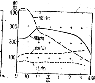
第55図 10月の末 晴れた日 東、西、南、北向きの各教室 の時刻による照度の変化の例
