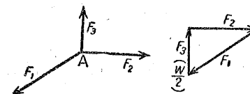
第39図 A点に働く力
