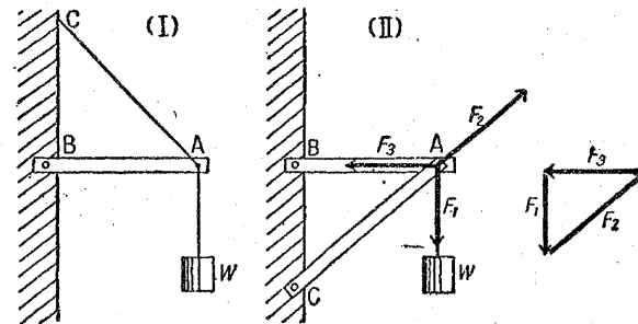
第43図 一端が自由なはりの補強
