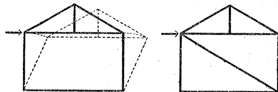
第44図 筋違のはたらき
