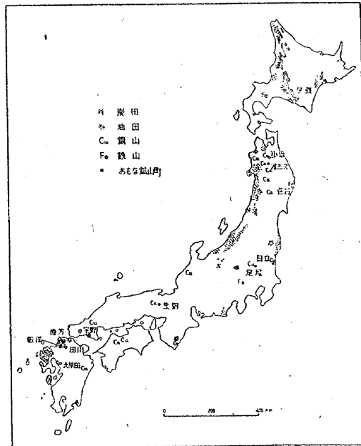
第 18 図 わが国のおもな鉱産分布
