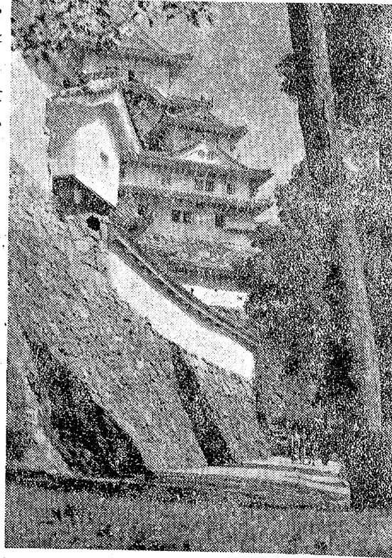
第 24 図 古城のおもかげ よって作られた美しい都市の風景である。
