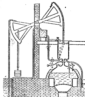
ニューコメンの大気圧機関
