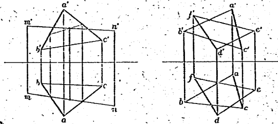
五 上ノ右ノ投影圖ハ、二ツノ三角形 ABC, DEF ヲ示シタモノデアル。ソノ交線ヲ求メヨ。
