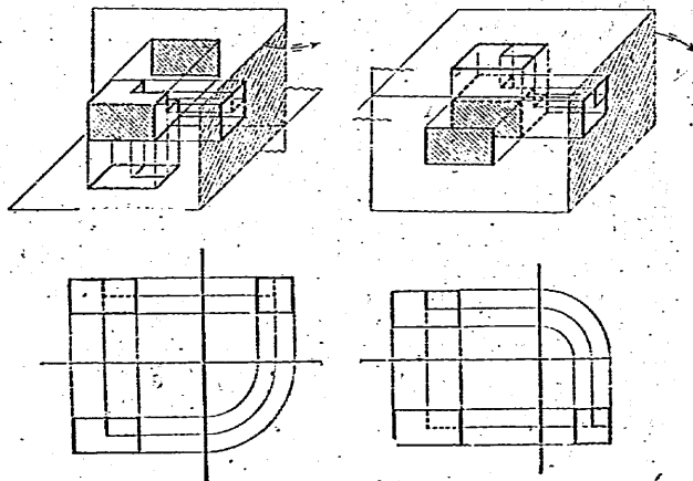
上ノ左ノ圖ニ示シタヤウナ三面圖ノ書き方ヲ 第一角法 トイヒ、右ノ圖ニ示シ
