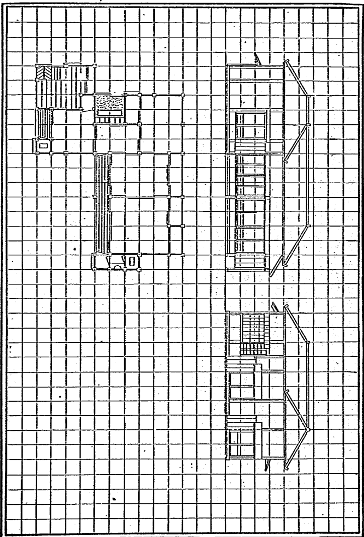
課外 瓦葺住宅の工作圖
