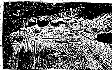
スイスたるては被に河水で會、痕擦の河水石の圓で痕擦河水るゐてつ殘に方地ンルツルの塊石たれら削の角稜に爲の動移りま拔に底河水は
