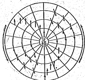
てつ向に北は又南 化變の向風 図 る變が向方に第次く如の圖は風く吹
