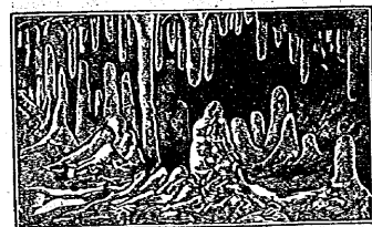
石乳や石筍が群立する 洞内の石灰洞部
