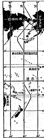
體大 線更變附日(註) 基に線經の度十八百は がるみてつなにとく 上宜便で等係關の土領 るおも處ためしせ曲屈
