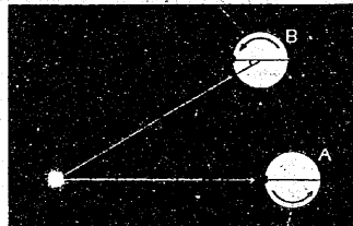
A、つし轉自が球地 日陽太と日星恆(註) 分幾向に上たし轉自一とるす轉公にBらかいなし中南に點の元は陽太ばれけなら廻か
