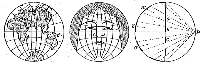
るなく狭は積面の心中でのたし寫透を側裏て立を板子硝に心中の儀球地 法圖射平儀圖
