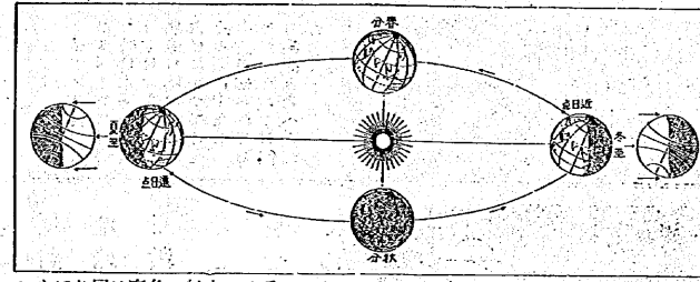
四季の起る理に節季より太陽の高さや之を受けける射角の度にてい
