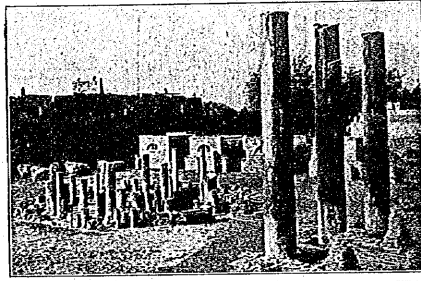
海後築建 址遺の堂スピラセるかに岸海のヤリタイ 隆起の痕跡の貝孔穿に部下の柱でのたし起隆又み沈に
