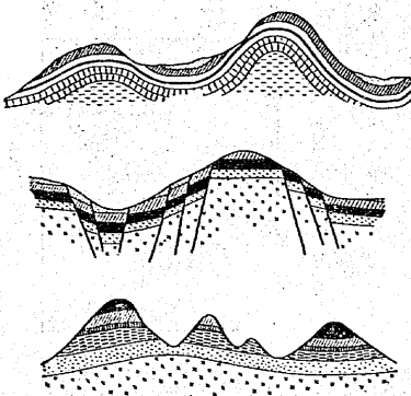
に層断は④りよに曲結は② 面断の岳山図 面断の脈山た來出りよに蝕侵の水流は①りよ
