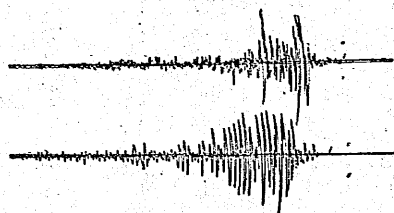
し壊破く悉は計震地たつかに京東 録記の震地東關圖殿山向の震仙は圖のこ たつかなら得を録記な全完て倍五・三約の圖のこは動實で動震たじ感に計震地の所象
