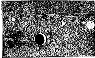
図1 星の運行の図 恆星・遊星・衛星の關係を示す
