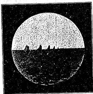
橋に僅は船の方遠 船た見らか岸海 ④ 見えが體全は船い見えが分部一の頭
