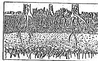
物機有に最多は層上 用作の根の物植 多に合割が物合混は層中 塊土るゐてじ混をるゐで石岩な質堅は層下 壤土強いなく
