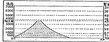
高度と气压の関係
