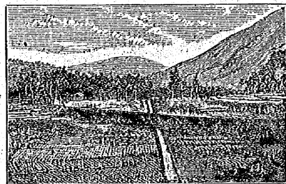
層斷大た米田に谷尾根の縣卓岐際地震尾浪 層斷圖も最は軒一約の近附谷尾根に殊び及に軒十六約が長延はたし動移を弱米三にも平水・米六がひ違喰の直垂くし其
