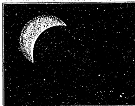
影の球地たつ映に面月際 ② の食月 ③
