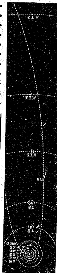
星のす属に系陽太陽西
