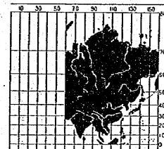
し等もで處何は隔間との線緯と線經 法圖ルートカルメ器圖 るなく長に第次てつ從にくづ近に極は隔間との線緯と線緯く
