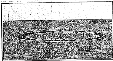
例一の礁環珊瑚あるに中の島群洋南 礁珊瑚
