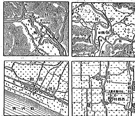
各圖の聚落の種別 ① 散村 ② 集村 ③ 山村 ④ 市街 ⑤ 市街 ⑥ 市街 ⑦ 市街 ⑧ 市街 ⑨ 市街 ⑩ 市街 ⑪ 市街 ⑫ 市街 ⑬ 市街 ⑭ 市街 ⑮ 市街 ⑯ 市街 ⑰ 市街 ⑱ 市街 ⑲ 市街 ⑳ 市街 ㉑ 市街 ㉒ 市街 ㉓ 市街 ㉔ 市街 ㉕ 市街 ㉖ 市街 ㉗ 市街 ㉘ 市街 ㉙ 市街 ㉚ 市街 ㉛ 市街 ㉜ 市街 ㉝ 市街 ㉞ 市街 ㉟ 市街 ㊱ 市街 ㊲ 市街 ㊳ 市街 ㊴ 市街 ㊵ 市街 ㊶ 市街 ㊷ 市街 ㊸ 市街 ㊹ 市街 ㊺ 市街 ㊻ 市街 ㊼ 市街 ㊽ 市街 ㊾ 市街 ㊿ 市街
