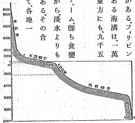
るめ占を部大が地臺海深く狭は帶沒陥・棚陸 斜傾の底海
