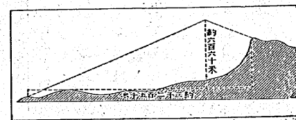
山に俄は山梯磐小る餘に米百六拔海 裂破の山梯磐 なるめてつ残てつなに形蹄馬が跡のそし散飛を分部大の體
