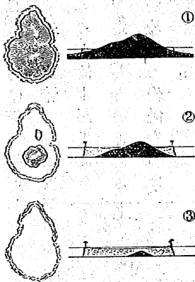
に狀形は礁珊瑚 類種の礁珊瑚 如の①のりけ分に種三てつよ 如の②のいといと礁環をのゐてし着附をのむ圍を地陸でん換を水の帯一く海でしなを狀環く如の③のいといと礁堡別の等此 ふいと礁環をのむ圍を水の地土たゐてつ作を礁環はる來出のれはいとるゐて爲たし降下に第次
