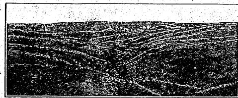
形地の期年幼図 るあて調平に體全が貌地で慢緩てし概が伏起
