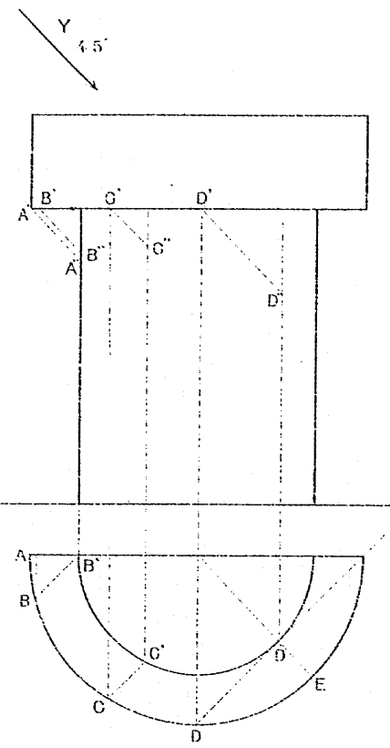
甲 圓板ヲ戴ケル圓柱ノ陰影圖
