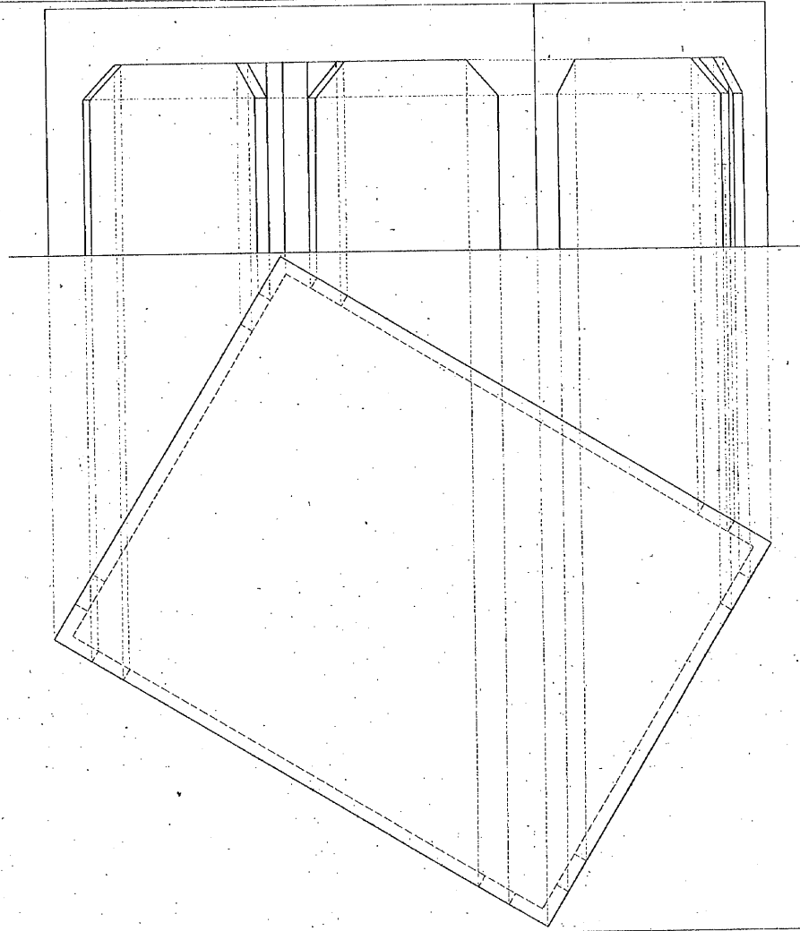
第十八圖 應用ノ二 札 縮尺十分ノ一
