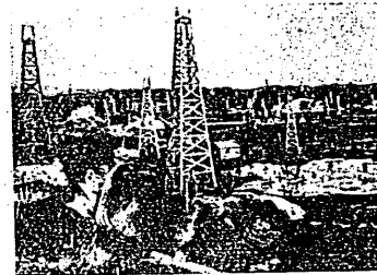
豊川油田
