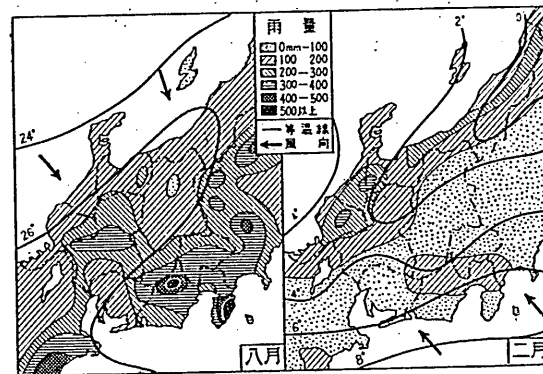
気象図
