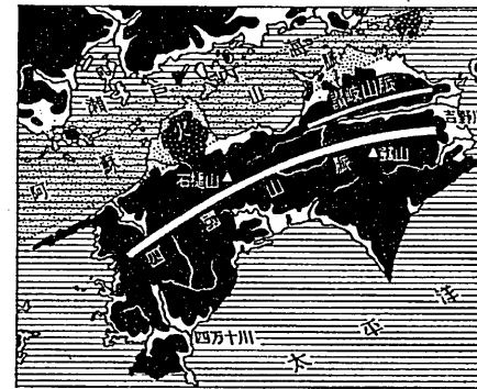
地形圖
