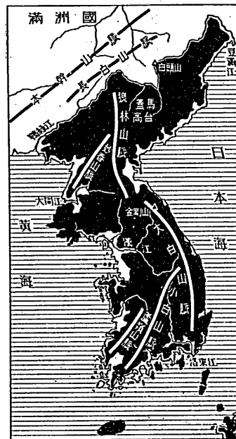
地形圖
