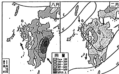
気象圖
