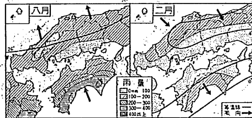
気 象 図
