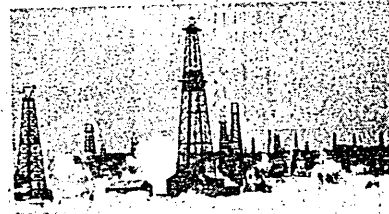
越後油田
