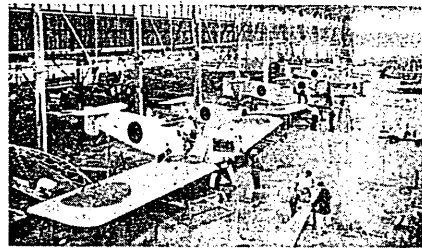
愛知時計電機株式会社飛行機組立工場
