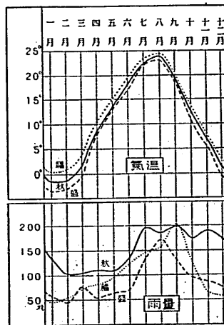
氣象圖
