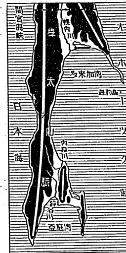
地形図
