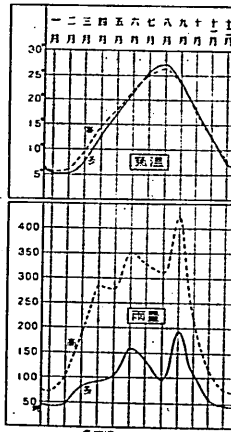
氣象圖
