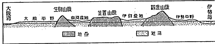
山形断面圖
