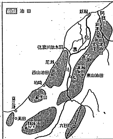
越後の油田
