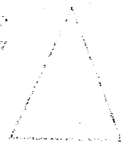
角三鏡
