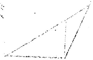
形三角
