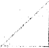
角三鏡
