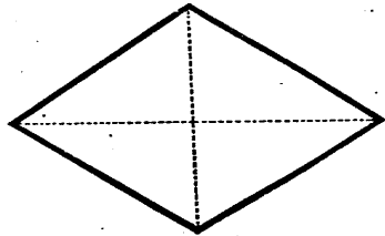
形方斜
