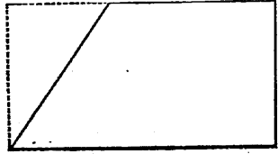
形梯
