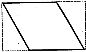
形方斜
