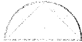
半圓
