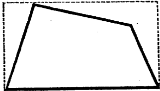
形邊四等不
