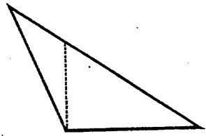
角三鏡
