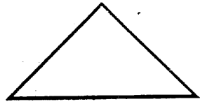
角三鏡
