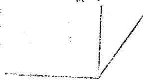
形三角
