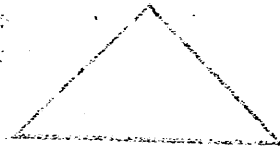
形三角
